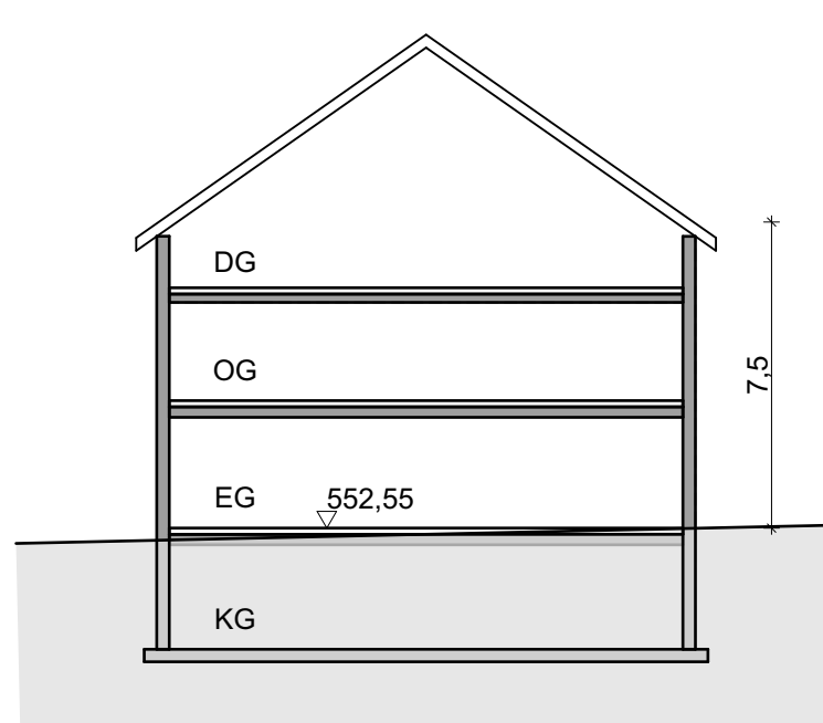
SCHEMASCHNITT NUTZUNGSCHABLONE 3 M : 1:200
